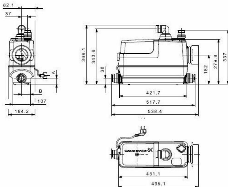
Рис. 27 Габаритные чертежи Sololift2 CWC-3
